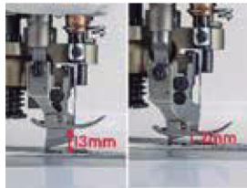
Acionador do calcador digital (sem solenoide)
