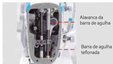
Sistema de barra de agulha livre de óleo
