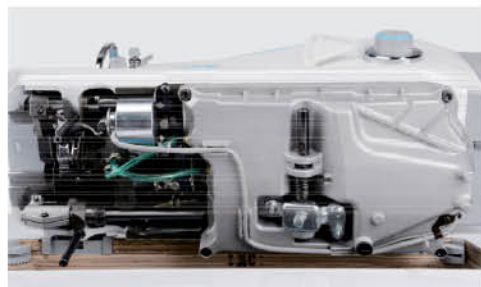
Cárter seco
